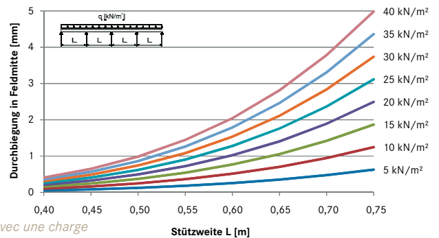
Flèche du panneau de coffrage K1 yellowplan Ép. = 27 mm
