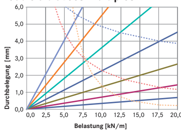
Poutre à travées multiples
