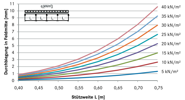
Flèche du panneau de coffrage K1 yellowplan Ép. = 21 mm
