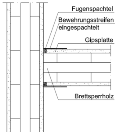
Abbildung 61: Anschlussdetail einer bekleideten Brettsperrholzwand in Anlehnung an [ÖNORM B 2320]
