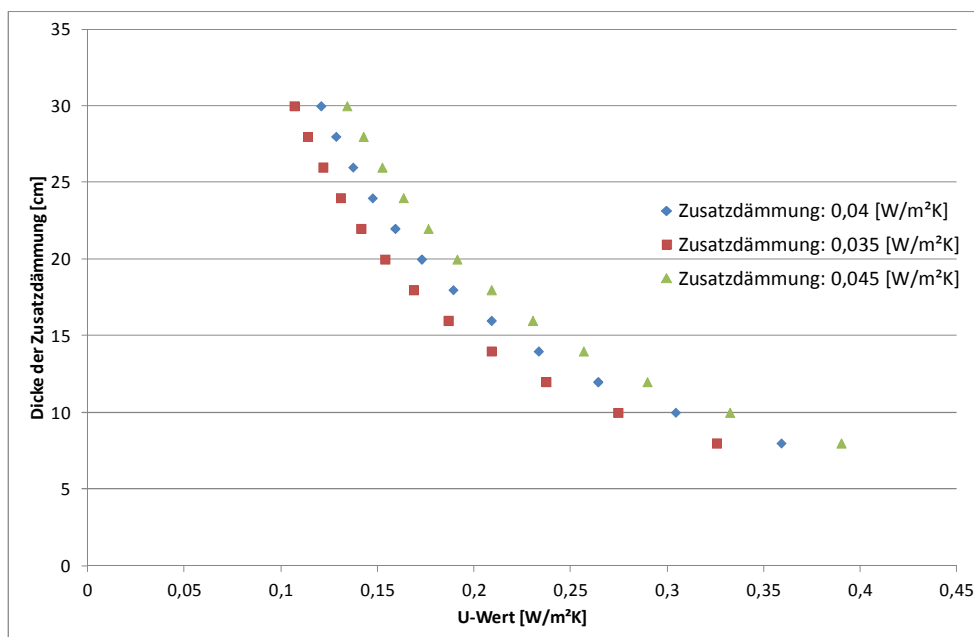
Abbildung 28: U-Werte einer 8 cm dicken Brettsperrholzwand ( \lambda : 0,13 W/m²K) in Abhängigkeit der Dicke und der Wärmeleitfähigkeit der Zusatzdämmung
