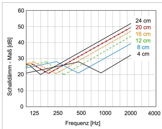
Abbildung 21: Berechnetes Schalldamm-Ma von fugenlosen Massivholzplatten in Abhangigkeit von deren Starke, Quelle: [Bednar et al. 2000]
