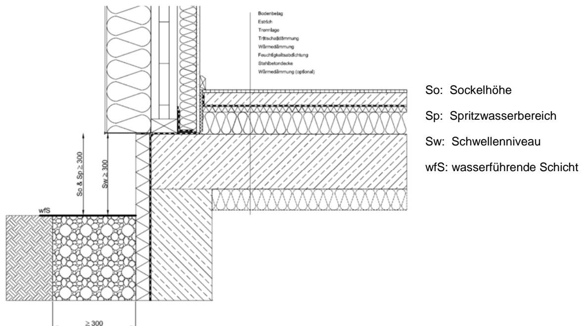
Abbildung 47: Standardsockeldetail Quelle:
