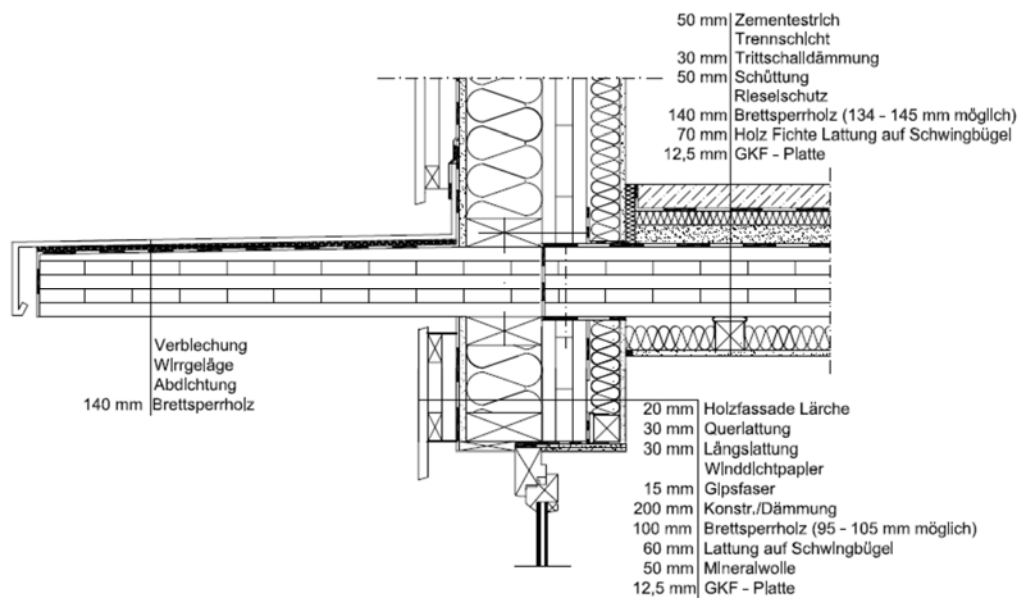
Abbildung 71: Beispielhafter Anschluss einer brandabschnittsbildenden Trenndecke an die Außenwand (80 cm „Auskragung“)
