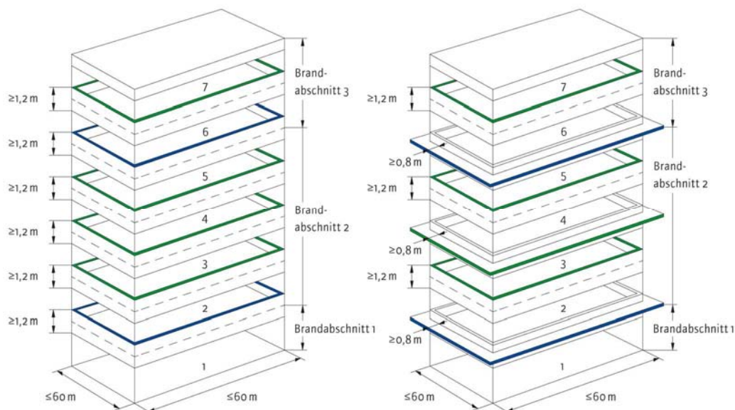
Abbildung 11: Anforderungen an Brandabschnitte und deckenübergreifende Außenwandstreifen bei GK 5 mit mehr als sechs oberirdischen Geschößen (nicht Wohngebäude) Quelle: proHolz/HFA
