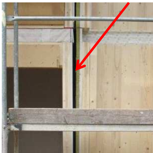
Abbildung 35: Steinwolle dämmung und unzulässige durchgehende Luftschicht zwischen Trennwand
