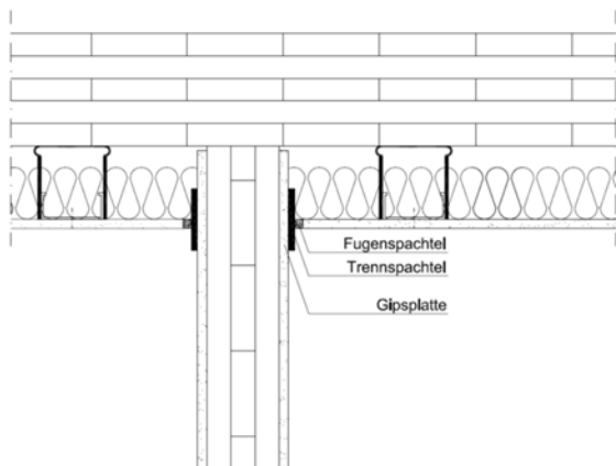
Abbildung 63: Anschlussdetail einer bekleideten Brettsperrholzwand an eine abgehängte Deckenkonstruktion in Anlehnung an [ÖNORM B 2320]
