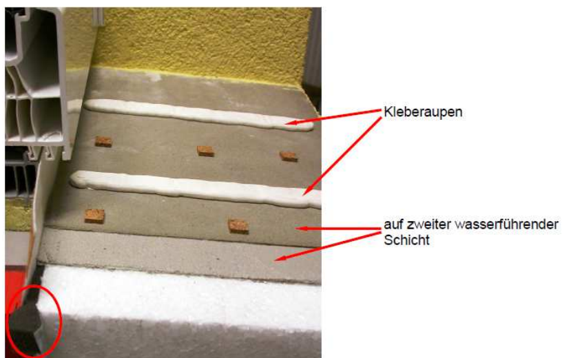
Abbildung 52: Fensterbankmontage auf zweiter Dichtebene mit Kleberaupen verklebt. Die dabei entstehenden Hohlräume sind zulässig. Der Anschluss des Dämmstoffkeiles / Fassadenplatte an das Fensterbankanschlussprofil erfolgt mittels Dichtband (roter Kreis). Quelle: [Österreichische Arbeitsgemeinschaft Fensterbank]
