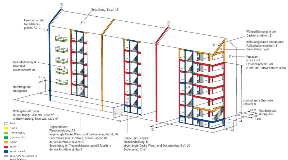
Abbildung 8: Anforderungen an den Feuerwiderstand und das Brandverhalten bei Gebaude der Gebaudeklasse 5, Quelle: proholz/HFA
