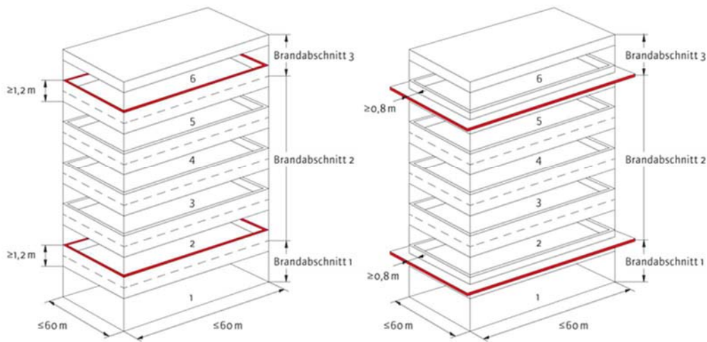
Abbildung 10: Anforderungen an Brandabschnitte und deckenübergreifende Außenwandstreifen bei Gebäude mit maximal sechs oberirdischen Geschößen (nicht Wohngebäude) Quelle: proHolz/HFA
