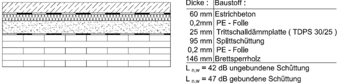
Abbildung 36: Einfluss der Schüttung auf den bewerteten Normtrittschallpegel L_{n,w} , Quelle: [Ferk 2006]
