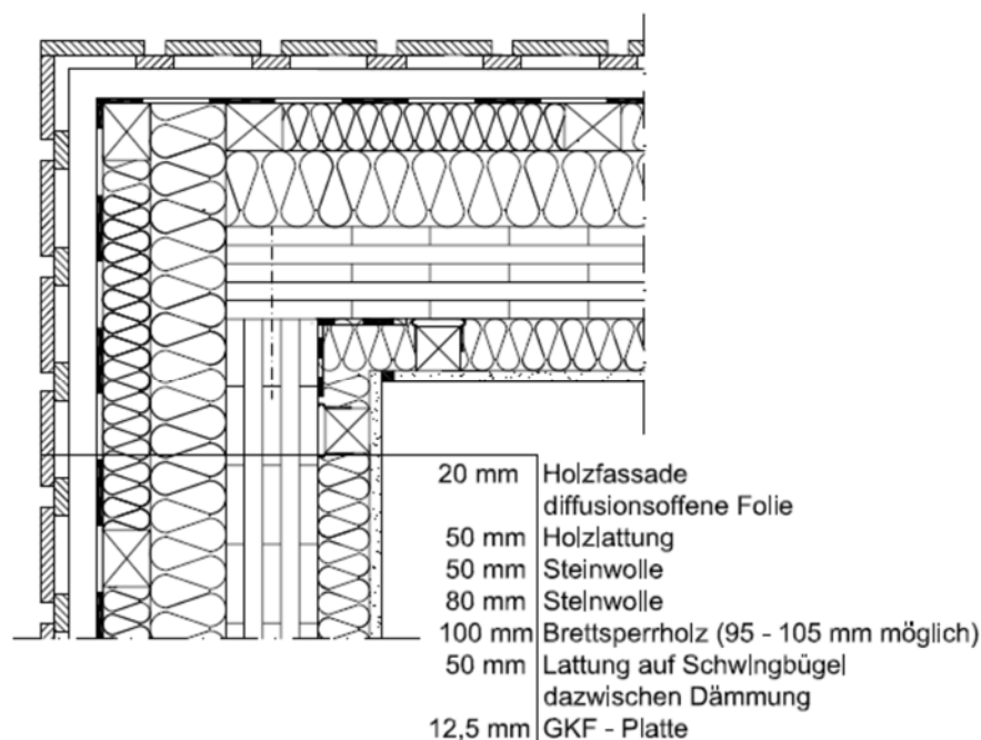
Abbildung 57: Beispielhafte Ausführung Außenwandecke mit Installationsebene
