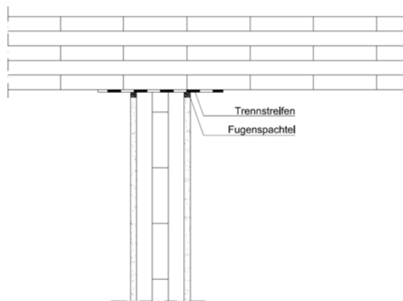
Abbildung 62: Anschlussdetail einer bekleideten Brettsperrholzwand an eine Deckenkonstruktion in Anlehnung an [ÖNORM B 2320]
